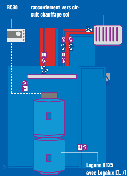
Logano G125 avec régulation EMS
